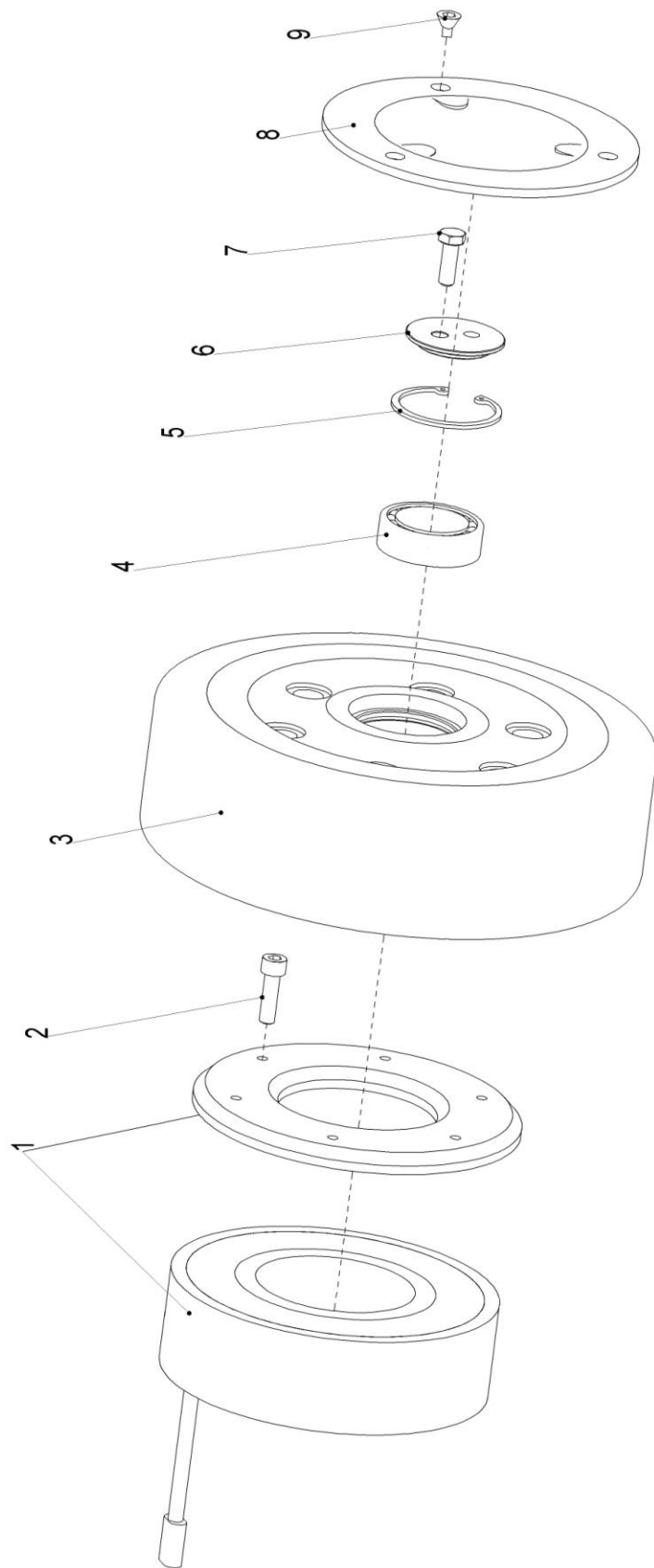
Fig. 7 Load roller
