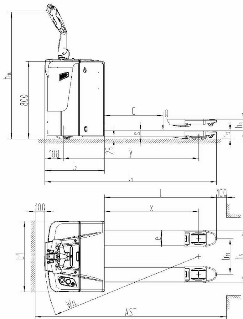
Рис. 2: Технические характеристики
